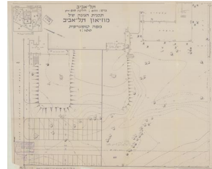
מפת מדידה של גן המוזיאון מ-1993, עם סימון טופוגרפי, מבנים ועצים בוגרים. מתוך הארכיון ההנדסי של עיריית תל אביב.
