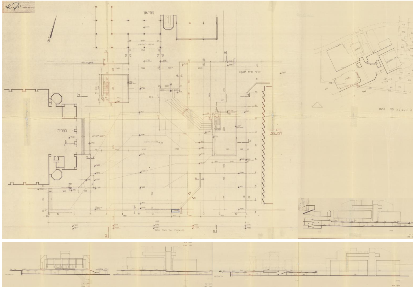
תכנית וחתכים של המרחב מ-1969. אדריכל יצחק ישר חתום על המסמכים. מתוך הארכיון ההנדסי של עיריית תל אביב
