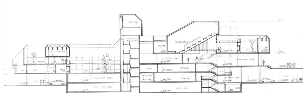
חתך. מימין ניתן לראות את החיבור לרחבה ואת החניון התת קרקעי. מתוך הספר "אחרי המודרניזם"
