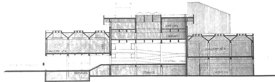
חתך אורכי. מתוך קטלוג תערוכת "הבניין: 50 שנה"
