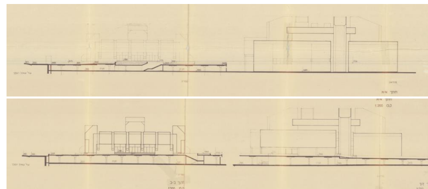
חתכים של המרחב מ-1969. מבנה המוזיאון והחניון שמתחת. מתוך הארכיון ההנדסי של עיריית תל אביב
