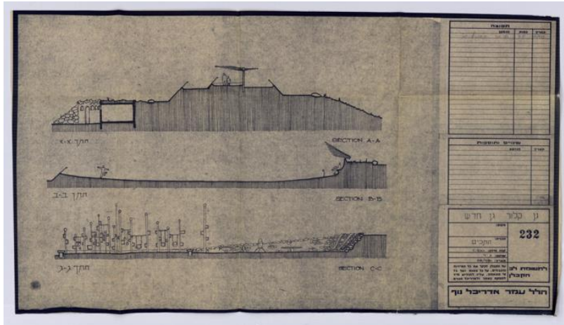
הלל עומר, חתכים, 27.10.1980, מתוך: ארכיון אגף שפ"ע
