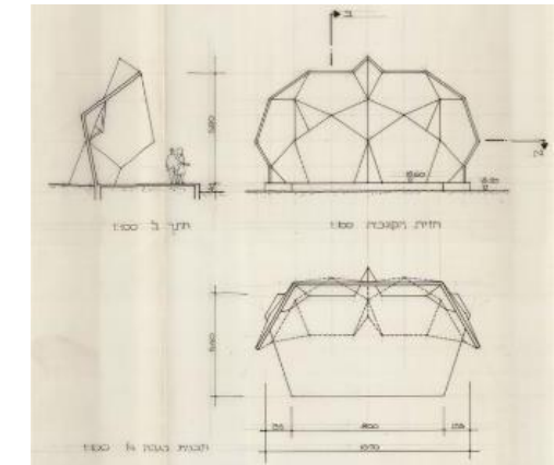
תכנית, חזית וחיתוך מתוך היתר הבנייה שהוגש לעירייה, אוסף אדר' צבי הקר
