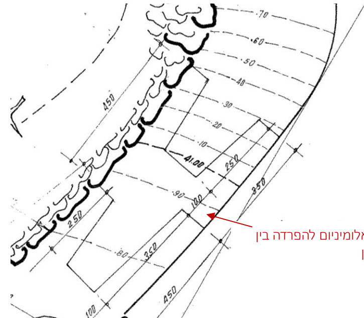
קטע מתוך תכנית כניסה מרח' הטייסים / לה-גרדיה, באדיבות משרד תכנון נוף בע"מ
