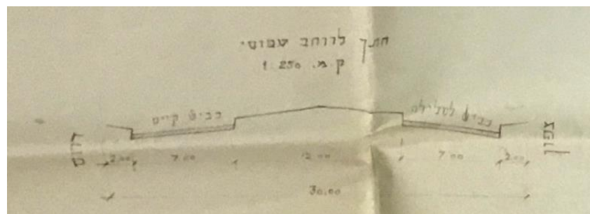
מקטעים מתוך תכנית שדרות החי"ל 1961 הכוללות גבהים, סימון צמחיה וחתכים עקרוניים, ארכיון אגף שפ"ע ערית ת"א-יפו
