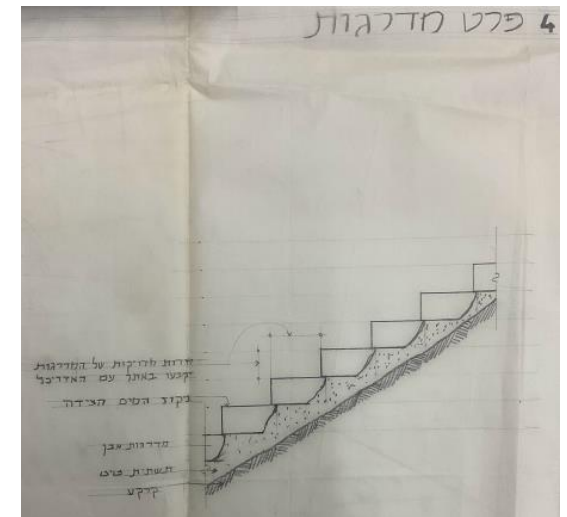
פרט מדרגות מתוך תכנית גן המדרון 1987 מתוך: אוסף סעדיה מנדל, ארכיון המרכז לחקר המורשת הבנויה בטכניון.
