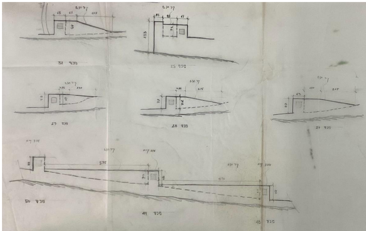
סקיצות לפריסת קירות ומיקום גופי תאורה בקיר, כלות לתכנית כללית לתכנית התאורה של גן המדרון משנת 1987
